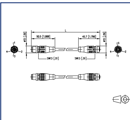
Schéma dimensionnel
