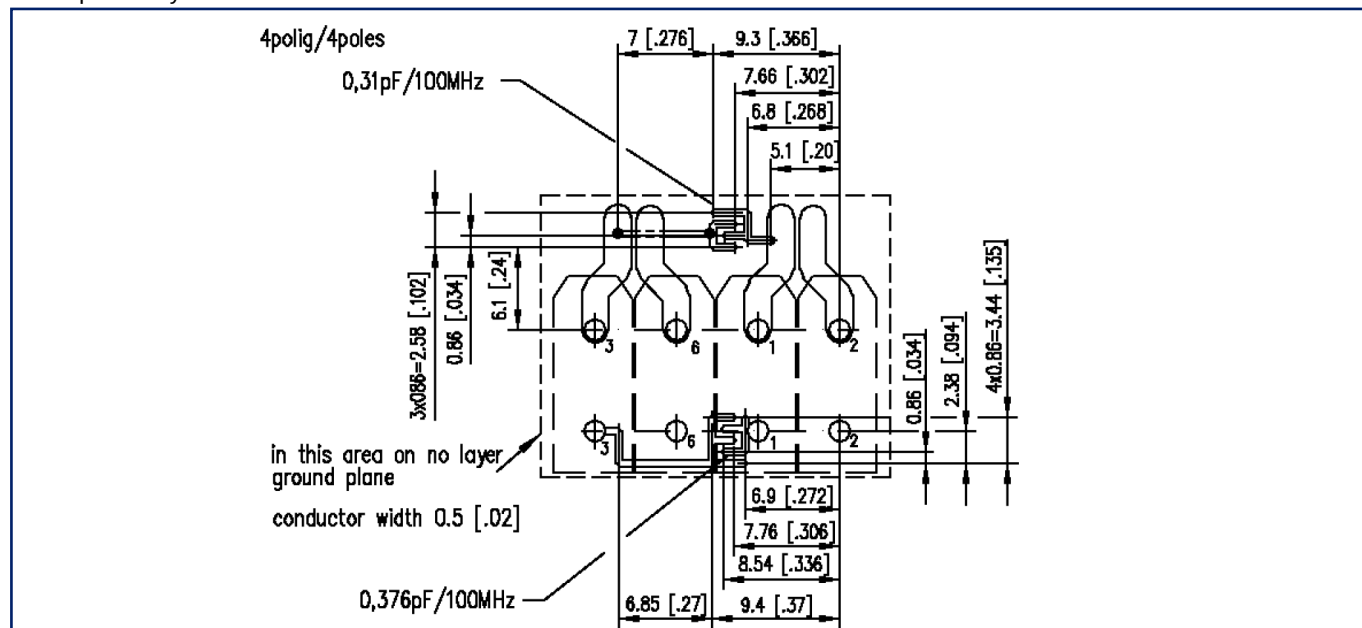
Leiterplattenlayout
