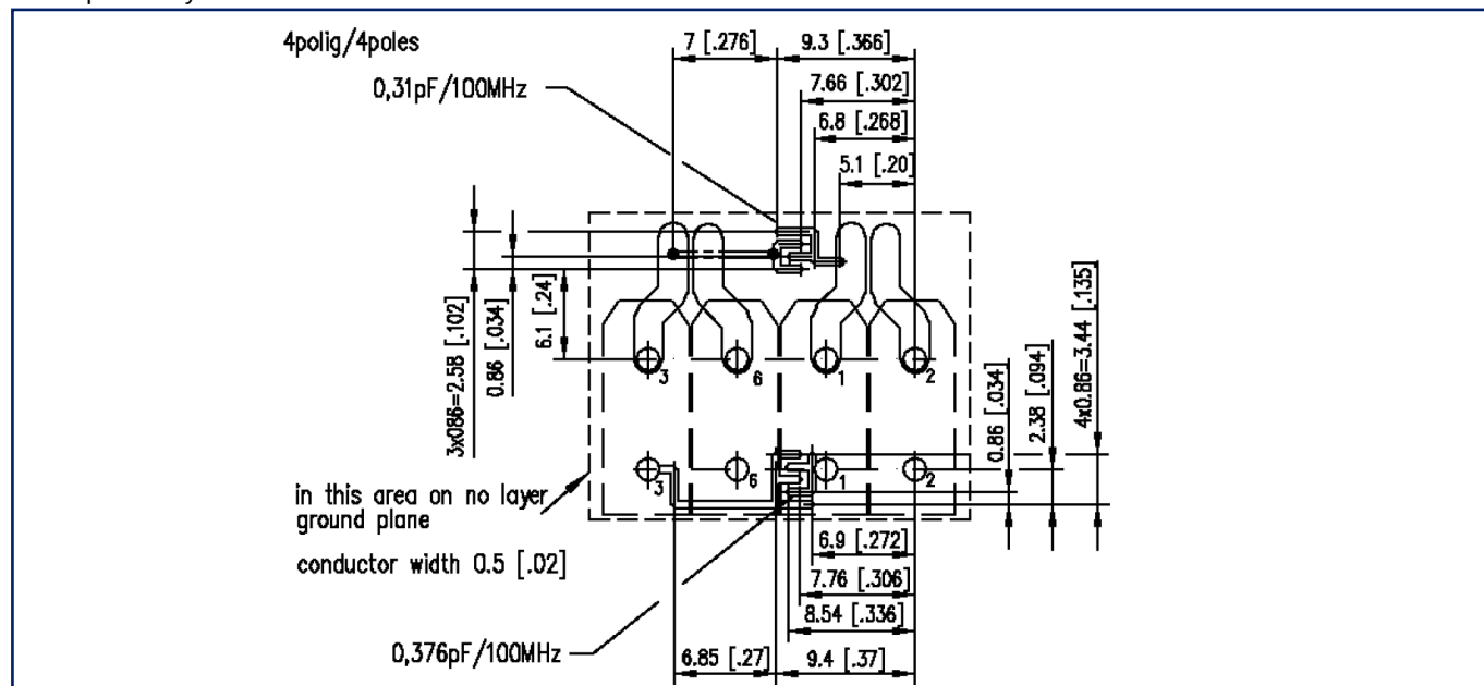
Leiterplattenlayout
