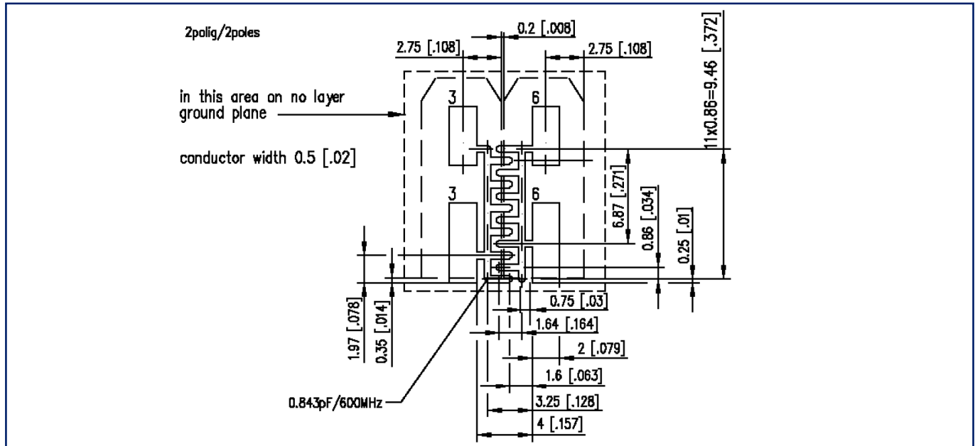
Leiterplattenlayout
