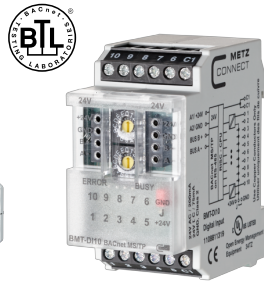
BMT-DI10
