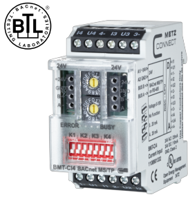
BMT-CI4
