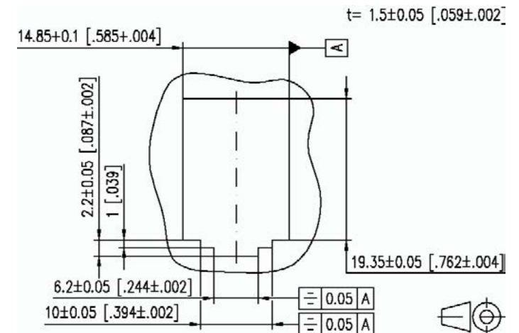
Masszeichnung MC Modul
