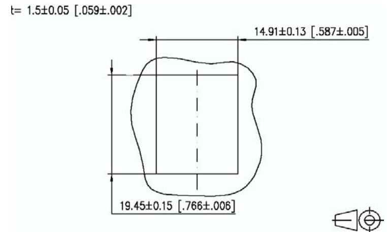
Masszeichnung Keystone
